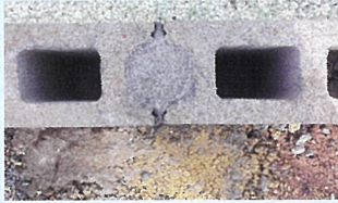
10cmブロックにフェンスの支柱(3.5cm×2.5cm)を立てる場合
